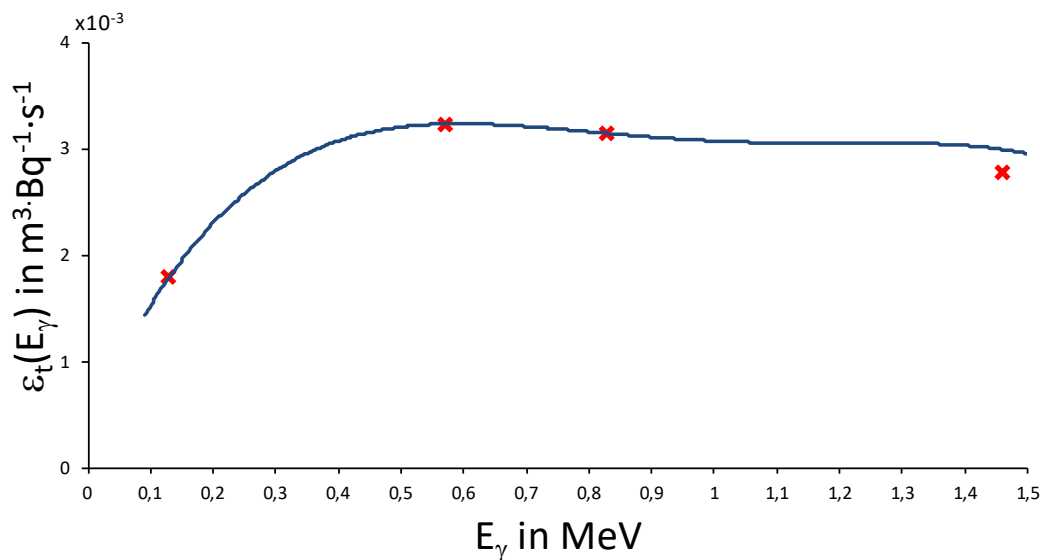
Abb. 3: Darstellung der verfahrensbezogenen, totalen Nachweiswahrscheinlichkeit \varepsilon_t(E_\gamma) für die Messanordnung „Sonde frei im Wasser hängend“.
