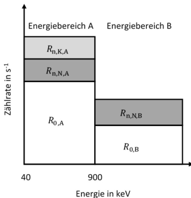
Abb. 4: Schematische Darstellung der Aufteilung der Gesamtbruttozählrate R_b im Gammastrahlungsspektrum auf zwei Gammastrahlungsenergiebereiche A und B
