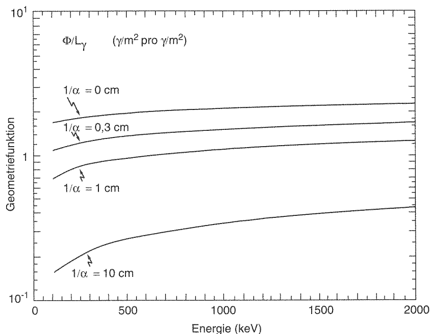
Abb. 3: Flußdichte der ungestreuten Gamma-Quanten im Energiebereich 100 keV bis 2000 keV bei Bodenkontamination unterschiedlicher Eindringtiefe ( 1/\alpha = 0 bis 10 cm). Zahlenangaben sind der Tab. 1 zu entnehmen
