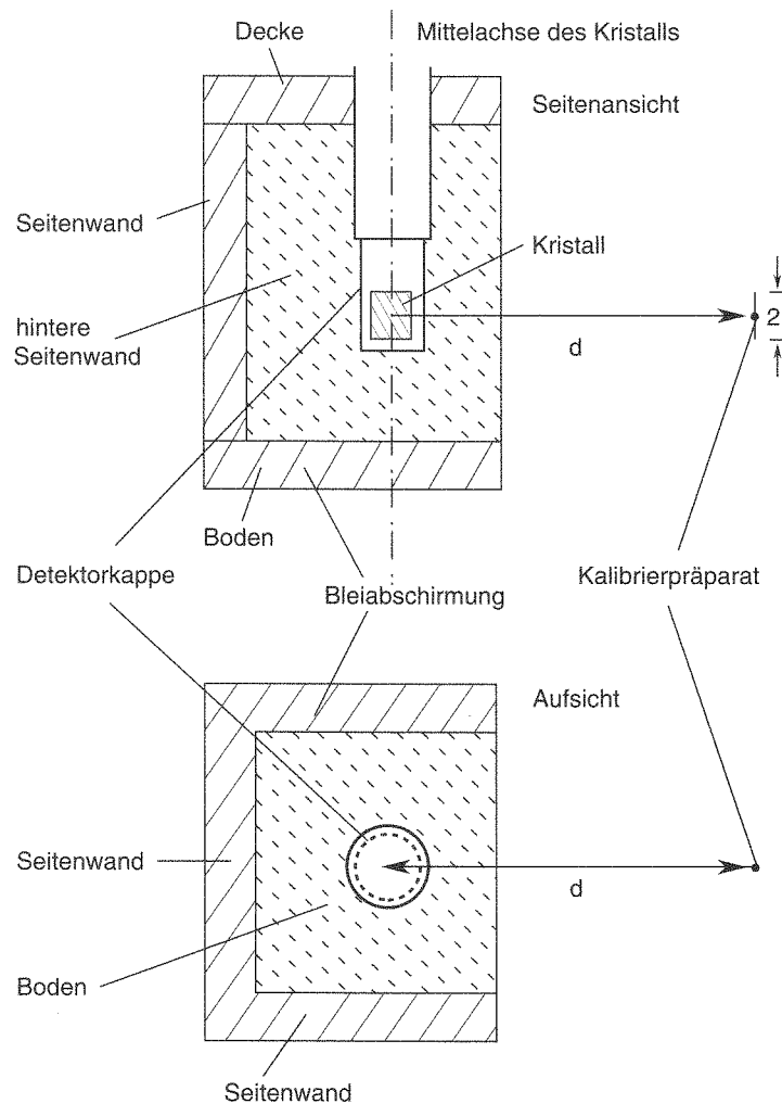
Abb. 2: Anordnung zur Kalibrierung des auf 5 Seiten mit Blei abgeschirmten Detektors. Der Abstand d = 1\text{ m} ist auf mindestens \pm 0,5\text{ cm} genau einzuhalten; die Abweichung 1 in vertikaler Richtung vom Kristallzentrum kann dagegen bis zu 5\text{ cm} betragen
