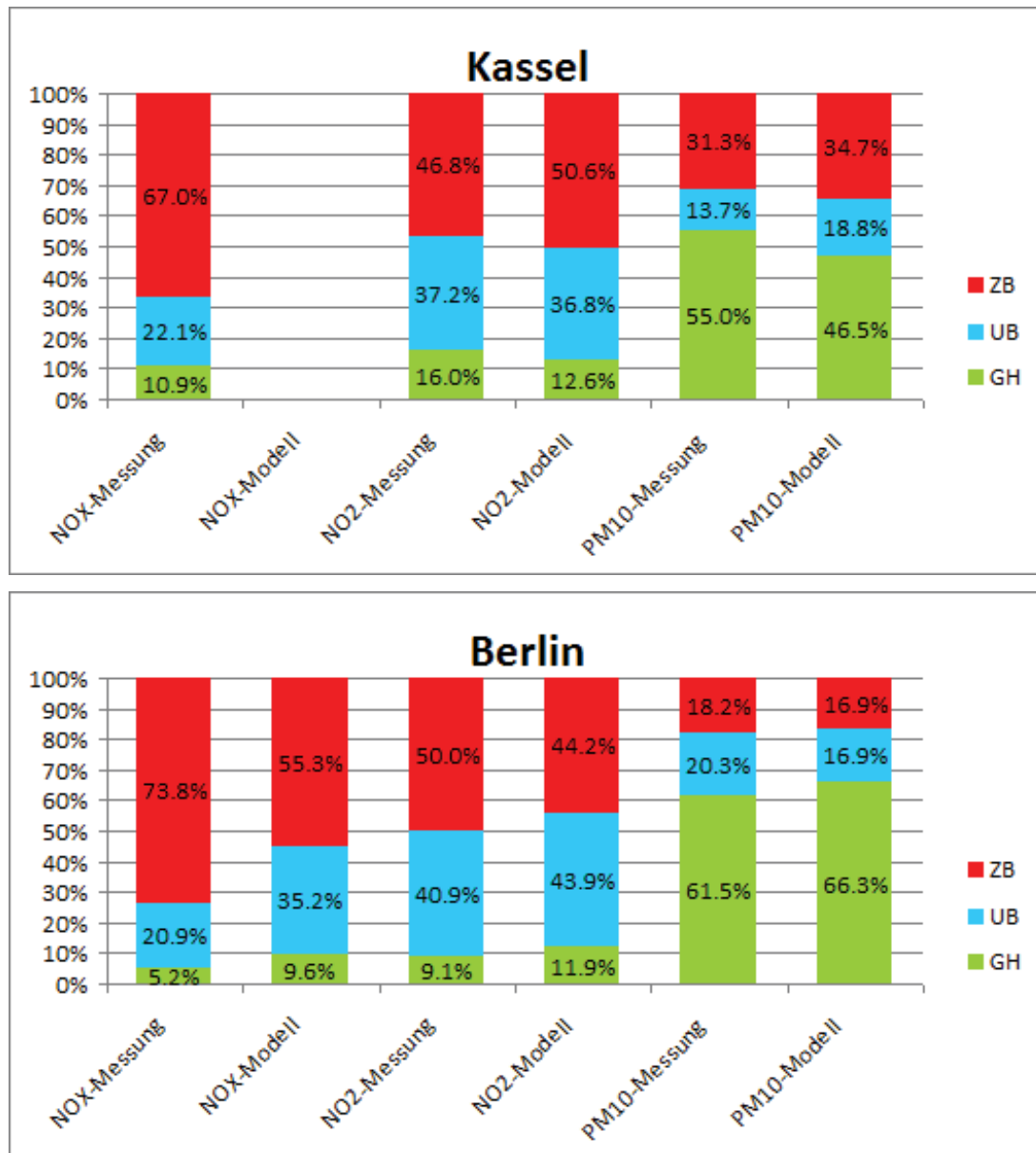
Abb. 33: Räumliche Verursacher im Vergleich von Modellrechnungen und Messungen in Kassel (oben) und in Berlin (unten)
