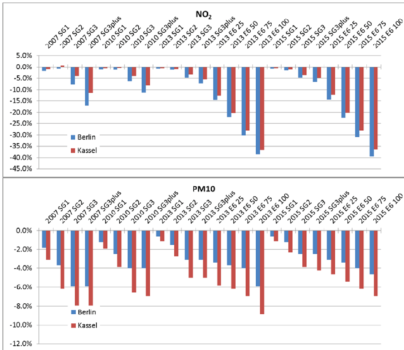
Abb. 36: Minderungspotenziale der Gesamtbelastung durch das Verbot verschiedener Fahrzeuggruppen bzw. den Ersatz durch Euro-6/VI-Fahrzeuge gegenüber der Basisberechnung im jeweiligen Bezugsjahr
