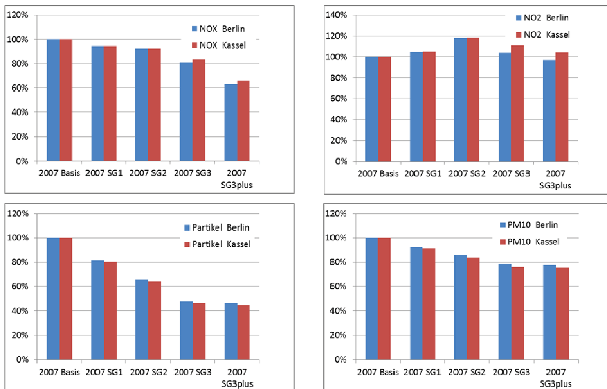
Abb. 34: Änderung der mittleren Kfz-Emissionen durch das Verbot verschiedener Fahrzeuggruppen bzw. den Ersatz durch Euro-6/VI-Fahrzeuge im Jahr der Einführung 2007
