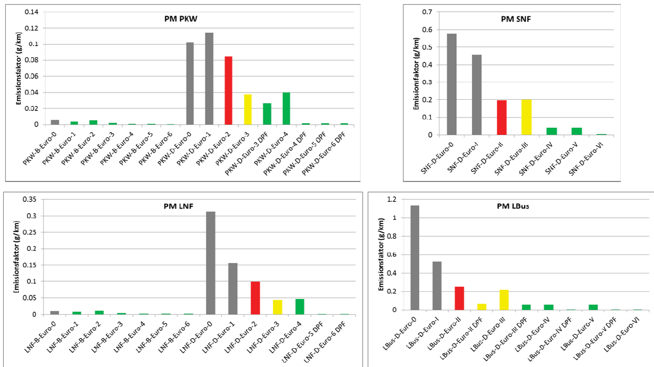
Abb. 31: Emissionsfaktoren nach Euro-Stufen für Partikel, unterschieden nach Pkw, leichten Nutzfahrzeugen, schweren Nutzfahrzeugen und Linienbussen. Auswertung auf Basis HBEFA 3.1 (INFRAS, 2010) für die durchschnittliche Innerorts-Verkehrssituation des HBEFA 3.1 im Bezugsjahr 2013
