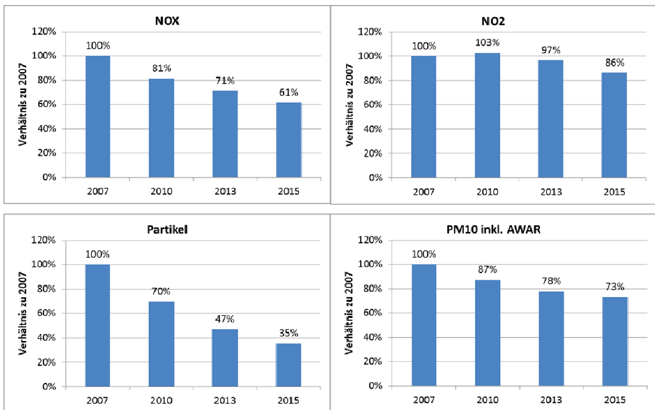
Abb. 32: Entwicklung der Emissionsfaktoren nach HBEFA 3.1 (INFRAS, 2010) am Beispiel der Verkehrsdaten der Frankfurter Allee in Berlin
