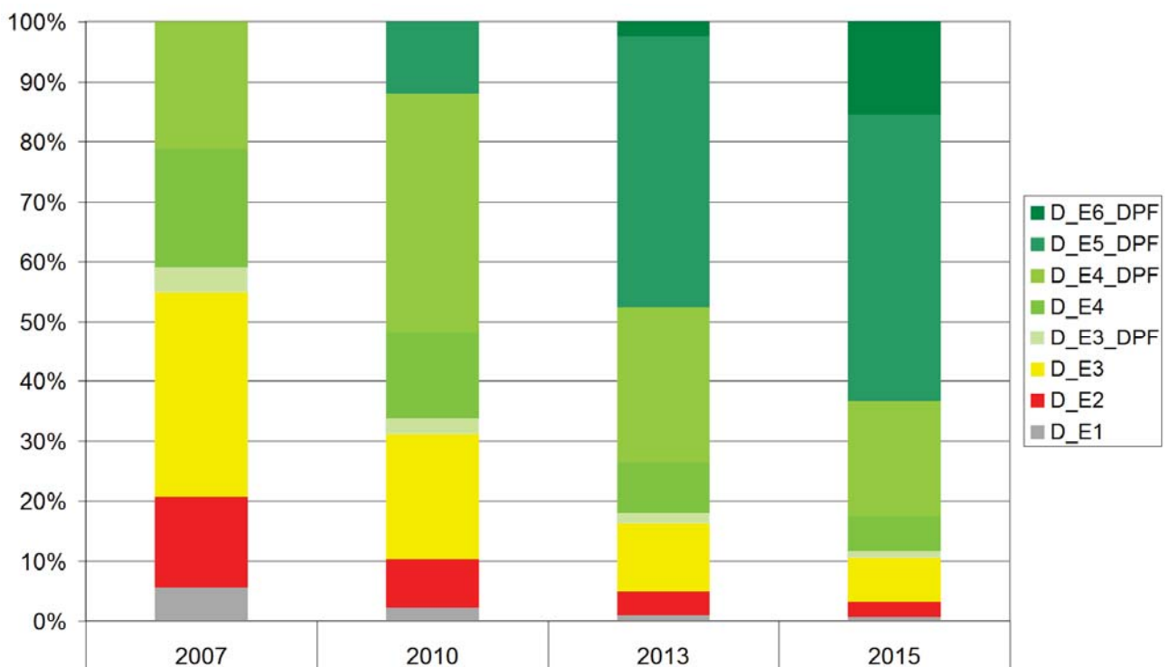
Abb. 28: Aufteilung der Diesel-Pkw-Flotte nach Euro-Normen getrennt nach Bezugsjahren nach HBEFA 3.1. Die Farben der Balken entsprechen der Farbgebung der Plaketten, wie sie zur Einfahrt in eine Umweltzone berechtigen, wobei grau für „ohne Plakette“ steht
