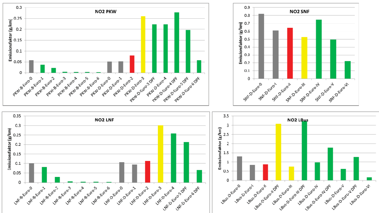
Abb. 30: Emissionsfaktoren nach Euro-Stufen für NO 2 , unterschieden nach Pkw, leichten Nutzfahrzeugen, schweren Nutzfahrzeugen und Linienbussen. Auswertung auf Basis HBEFA 3.1 (INFRAS, 2010) für die durchschnittliche Innerorts-Verkehrssituation des HBEFA 3.1 im Bezugsjahr 2013
