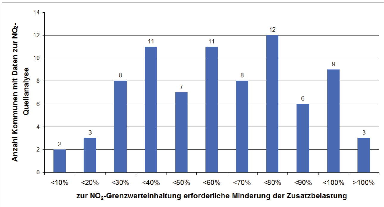
Abb. 40: Histogramm der zur \text{NO}_2 -Grenzwerteinhaltung erforderlichen Minderung der Zusatzbelastung in Kommunen, für die in den Plänen Daten zur räumlichen \text{NO}_2 -Quellanalyse aufgeführt wurden
