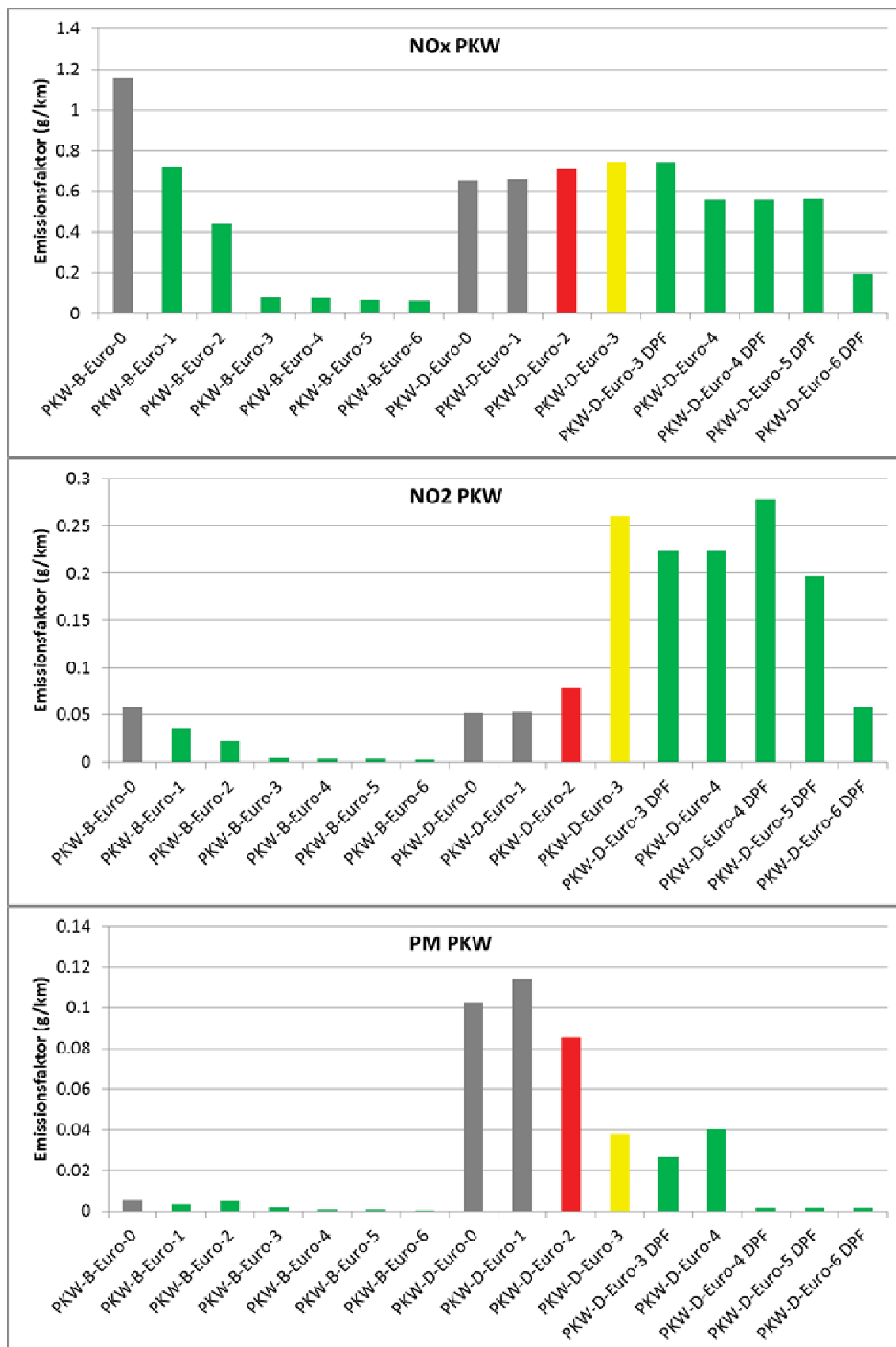
Abb. 27: Emissionsfaktoren für NO x , NO 2 und Partikel (PM) für Pkw getrennt nach den Euro-Normen und zusätzlich Partikel-filter nach HBEFA 3.1. Die Farben der Balken entsprechen der Farbgebung der Plaketten, wie sie zur Einfahrt in eine Umweltzone berechtigen, wobei grau für „ohne Plakette“ steht.
