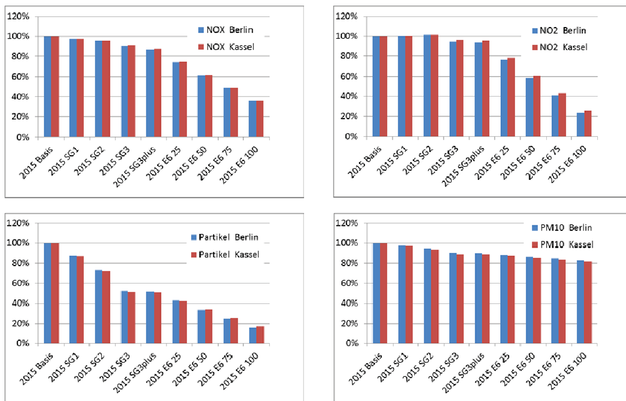
Abb. 35: Änderung der mittleren Kfz-Emissionen durch das Verbot verschiedener Fahrzeuggruppen bzw. den Ersatz durch Euro-6/VI-Fahrzeuge im Jahr der Einführung 2015
