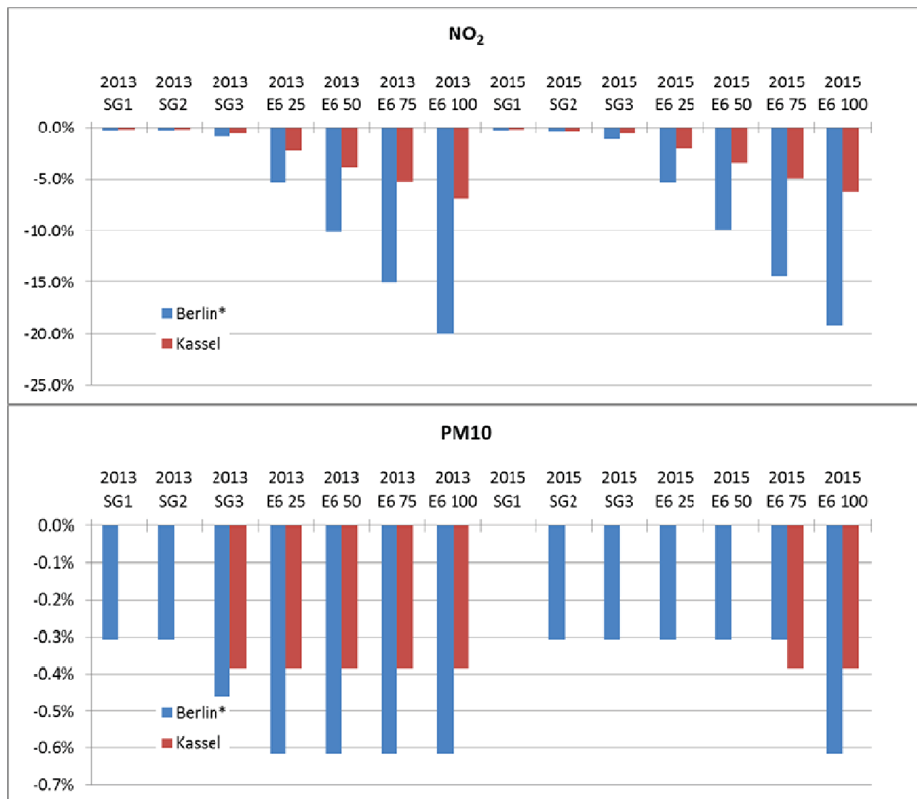
Abb. 38: Minderungspotenziale der Gesamtbelastung für die Erneuerung der Busflotte gegenüber der Basisberechnung im jeweiligen Bezugsjahr (*: Berlin mit angenommen Linienbus-Anteil von 6 %)
