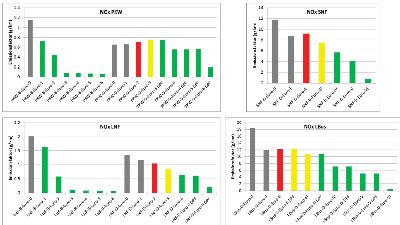
Abb. 29: Emissionsfaktoren nach Euro-Stufen für \text{NO}_x , unterschieden nach Pkw, leichten Nutzfahrzeugen, schweren Nutzfahrzeugen und Linienbussen. Auswertung auf Basis HBEFA 3.1 (INFRAS, 2010) für die durchschnittliche Innerorts-Verkehrssituation des HBEFA 3.1 im Bezugsjahr 2013
